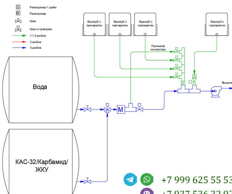
СХЕМА ВАРИАНТА КОМПЛЕКТАЦИИ
