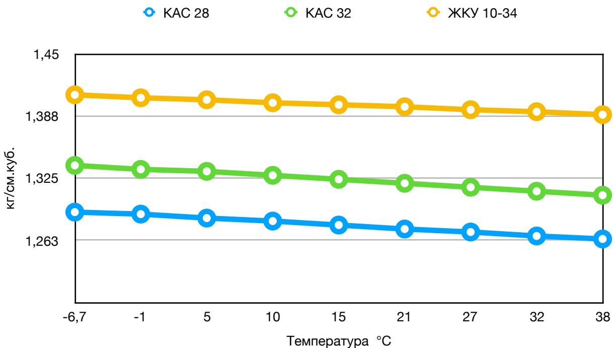
Изменение плотности растворов в зависимости от температуры.
